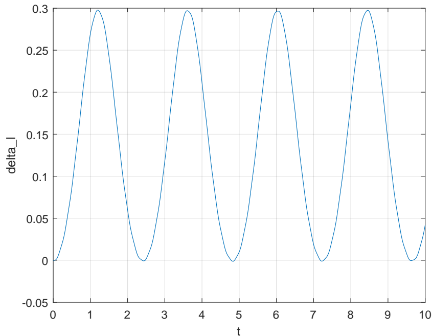
Abbildung 8: Federauslenkung
