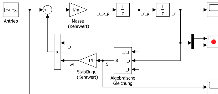
Abbildung 4: DAE-Blockschaltbild
