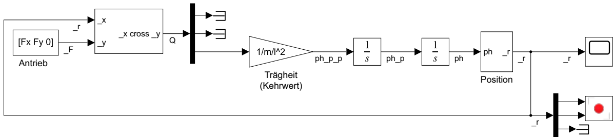
Abbildung 9: Polarkoordinaten-Blockschaltbild
