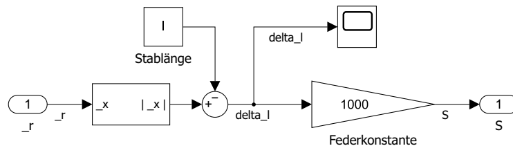
Abbildung 7: Stabfeder-Blockschaltbild
